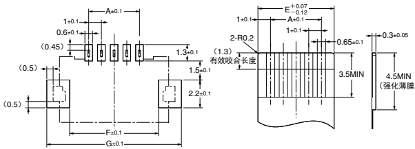
印刷基板加工尺寸 (顶视图)
